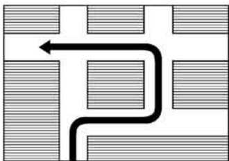
(Π - 6)
