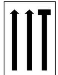
(Π - 70α)
