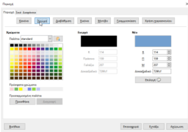
Εικόνα 4.15. Μορφοποιήσεις γραμμών
