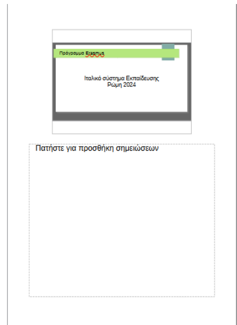
Εικόνα 4.25. Προβολή σημειώσεων
