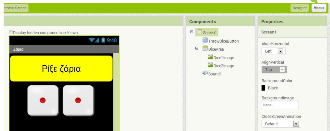
Εικόνα 12 - Κουμπί Blocks
