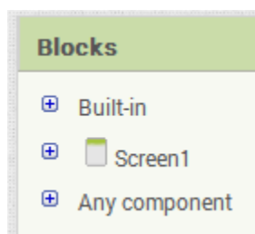
Εικόνα 14 - Ομάδες πλακιδίων
