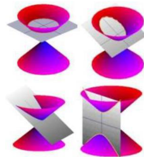
Γεωμετρικές Καμπύλες
