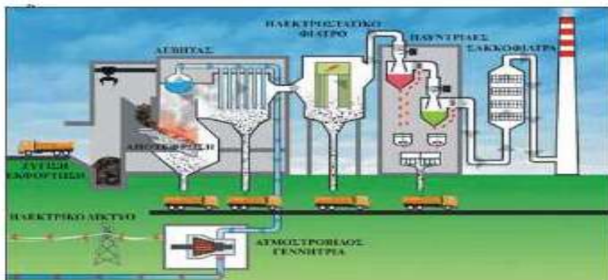
Εικόνα 1. Τυπική Μονάδα Αποτέφρωσης ΑΣΑ.( www.bsu.hr )
