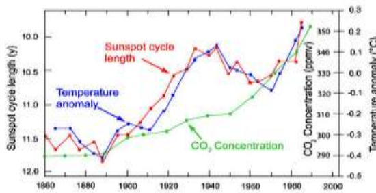
Εικόνα 4. Συσχέτιση των ηλιακών κηλίδων με την αύξηση της θερμοκρασίας και την συγκέντρωση του CO 2 στην ατμόσφαιρα. Friis Christensen, 2007.
