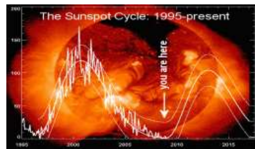
Εικόνα 5. Αριθμός των ηλιακών κηλίδων από το 1995 έως σήμερα. David Hathaway, 2008.
