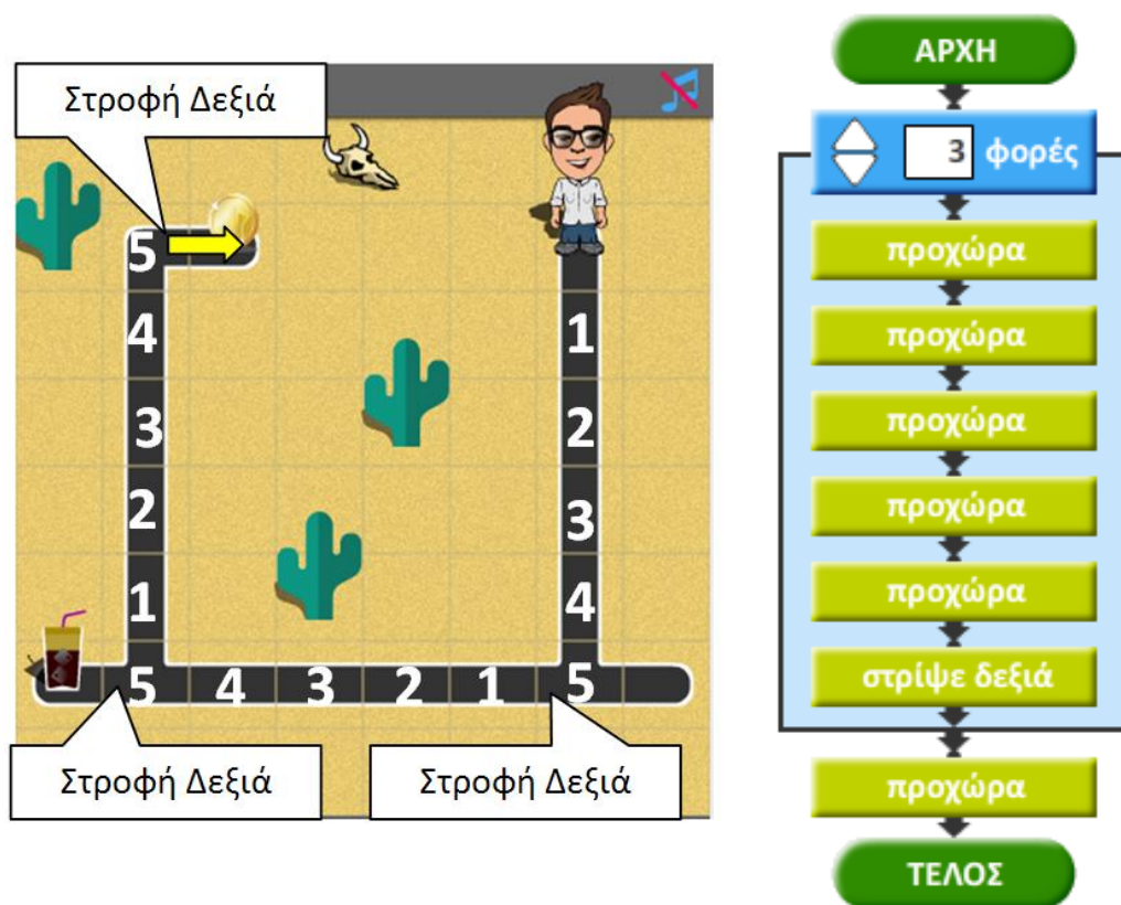
Σχήμα 3.18: Εικόνα παιχνιδιού και διάγραμμα ροής του κώδικα.
