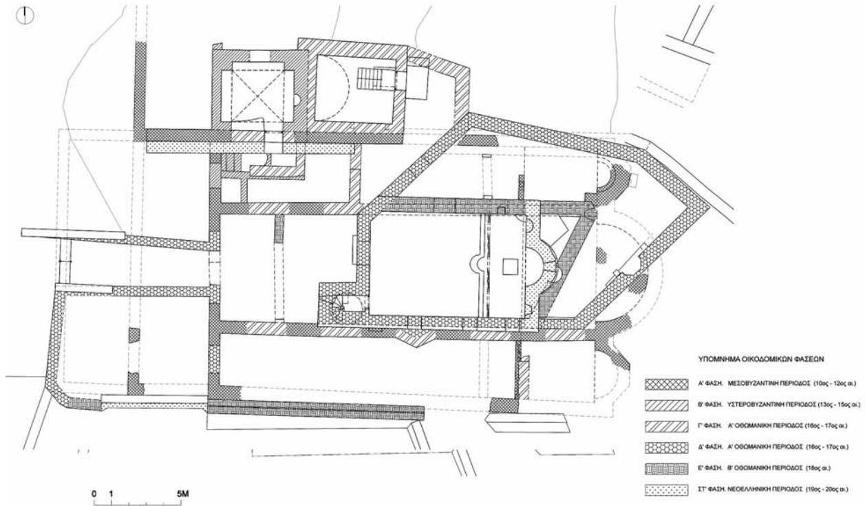
Σχ. 3. Ναύπακτος. Κάστρο. Ανασκαφή Προφήτη Ηλιού. Διάγραμμα οικοδομικών φάσεων.
