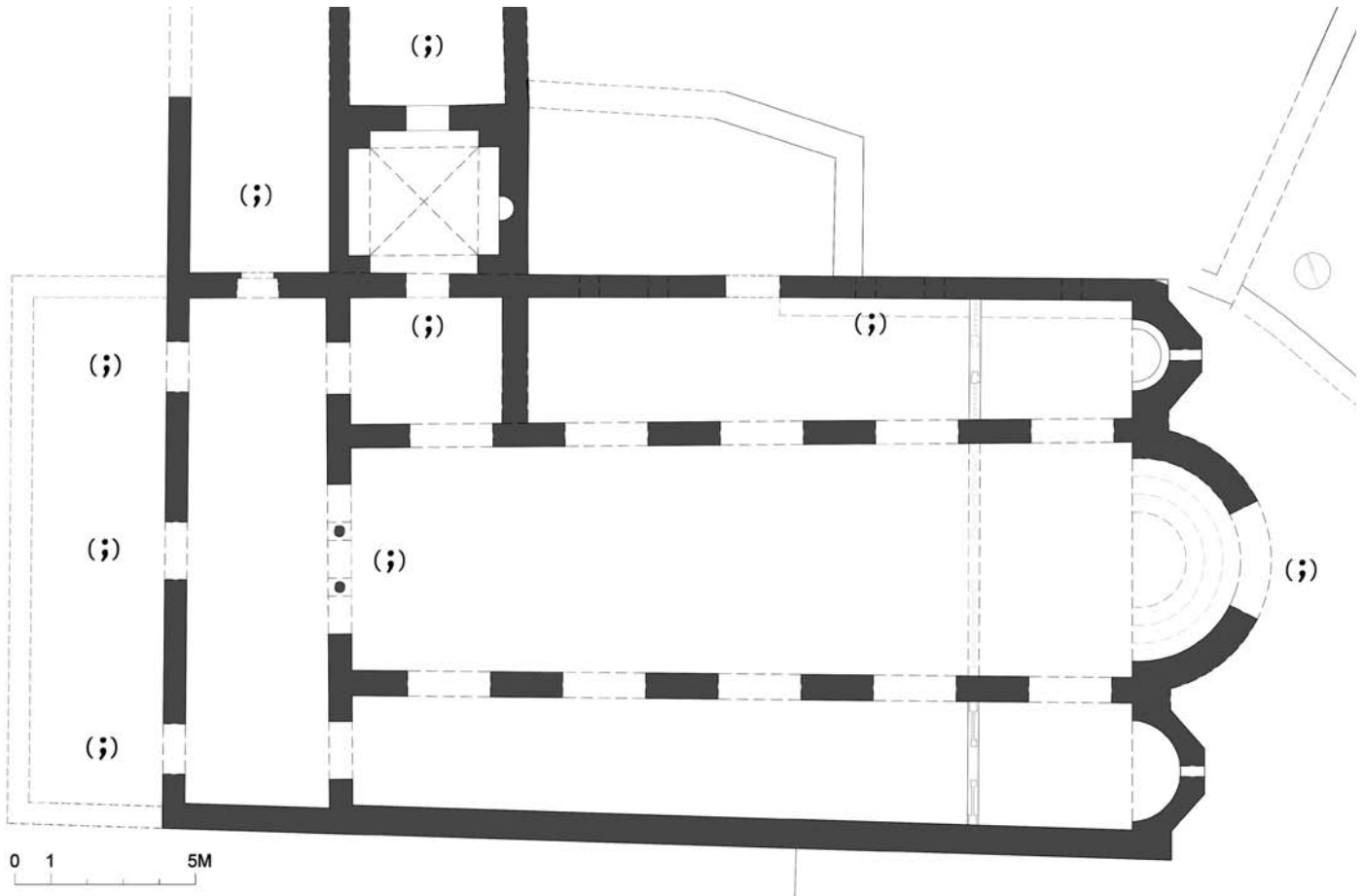
Σχ. 4. Ναύπακτος. Κάστρο. Ανασκαφή Προφήτου Ηλίου. Τρίκλιτη βασιλική. Αναπαράσταση. Κάτοψη.
