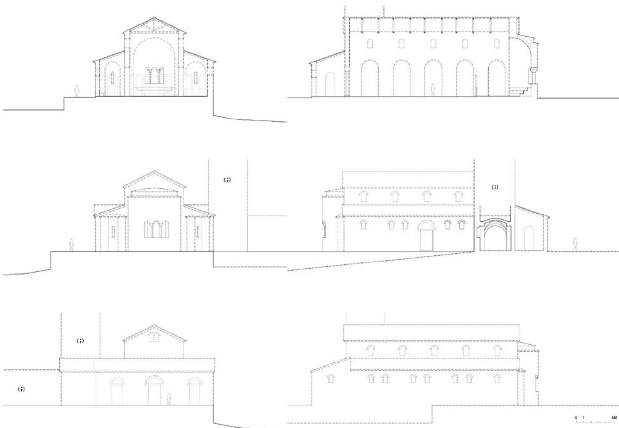
Σχ. 5. Ναύπακτος. Κάστρο. Τρίκλιτη βασιλική. Αναπαράσταση. Τομές και όψεις.
