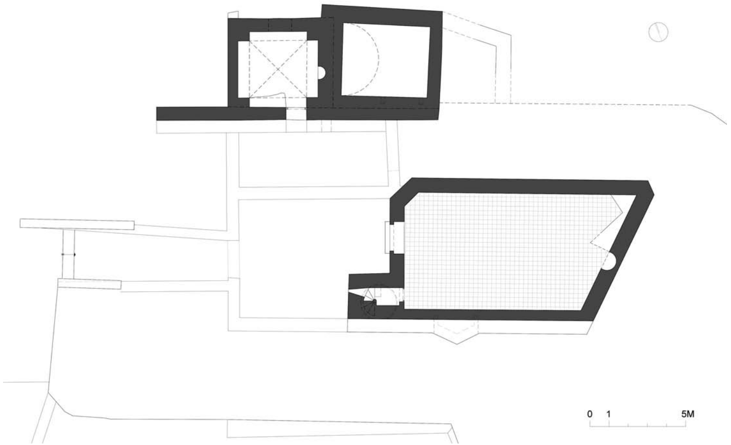
Σχ. 10. Ναύπακτος, Κάστρο. Τέμενος Γ. Αναπαράσταση: Κάτοψη.
