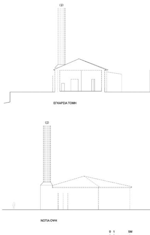
Σχ. 8. Ναύπακτος, Κάστρο. Τέμενος Β. Αναπαράσταση: Τομές και όψεις.
