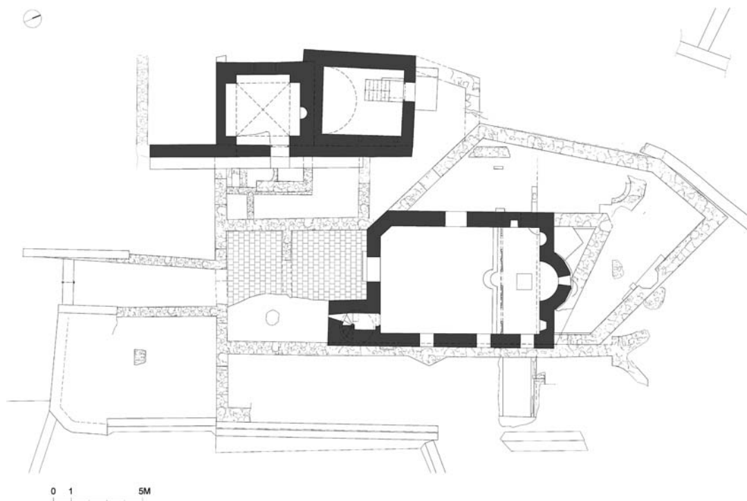
Σχ. 1. Ναύπακτος. Κάστρο. Ανασκαφή Προφήτου Ηλίου. Αποτύπωση. Κάτοψη.
