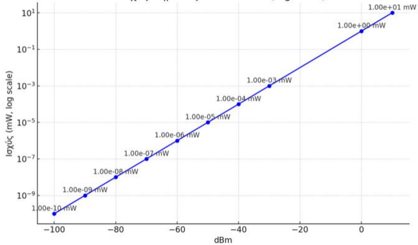
Ισχύς σήματος: dBm \leftrightarrow mW (log scale)
