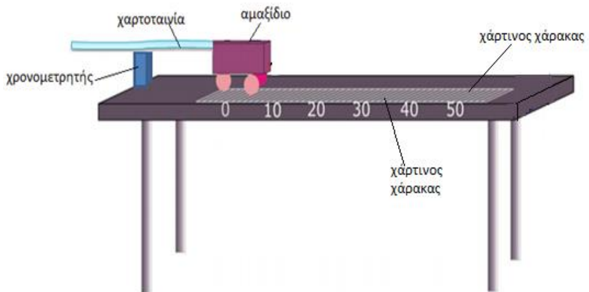
Σχήμα 1: Πειραματική διάταξη.
