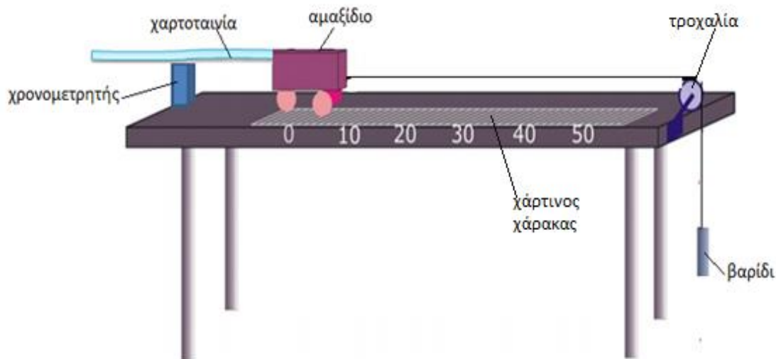
Σχήμα 1: Πειραματική διάταξη.
