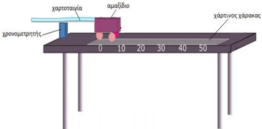
Σχήμα 1: Πειραματική διάταξη.
