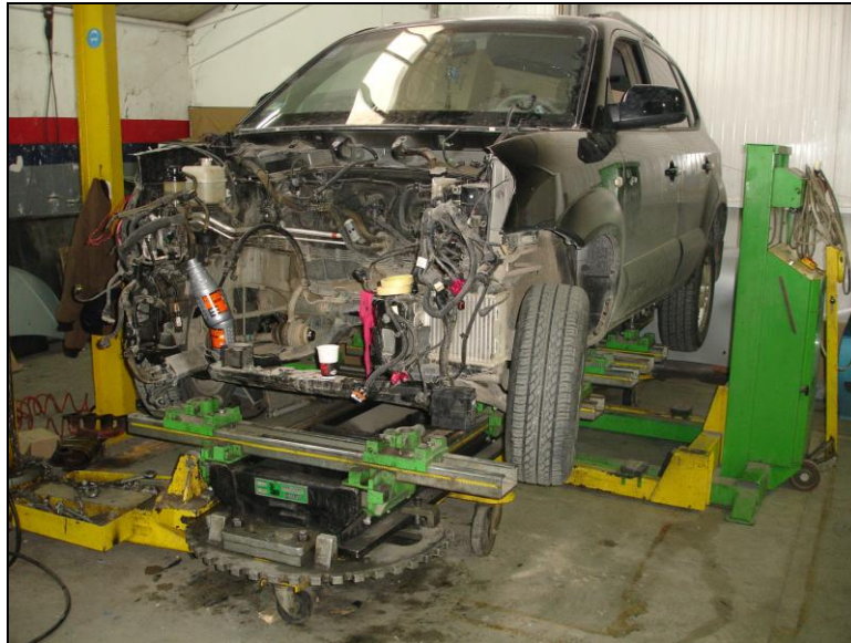
Εικόνα 29: Ειδικό μηχάνημα για την ευθυγράμμιση των αυτοκινήτων μετά από συγκρούσεις («καλίμπρα»).
