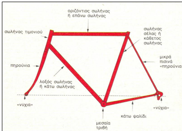
Εικόνα 75: Ορολογιακή σκελετού στο ποδήλατο (Πηγή: Wollzenmuller, F., 1984).
