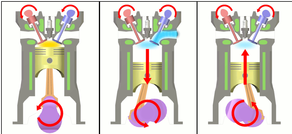
Εικόνα 2: Αρχή λειτουργίας τετράχρονου κινητήρα “Otto” (Πηγή: http://foter.com/Four-stroke-engine/ ).
