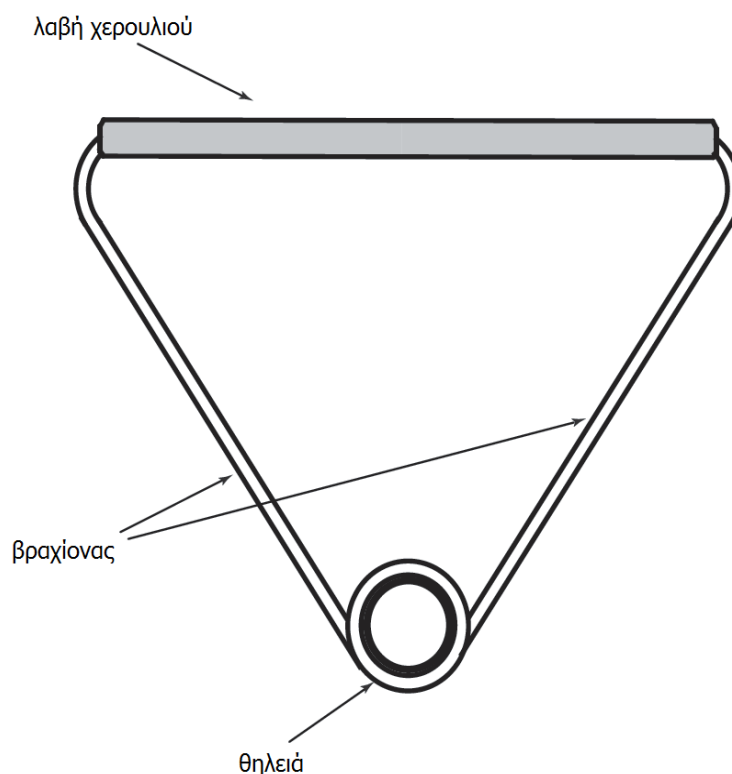
Σχήμα 191β: Γενική μορφή χερουλιού σφύρας
