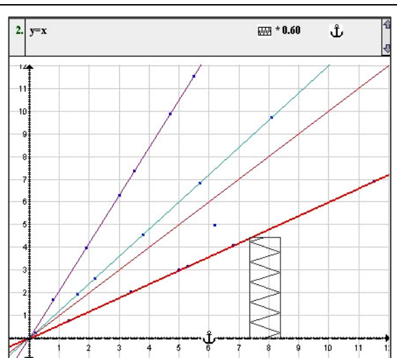
Εικόνα 35: Περιστροφές της y=x .
