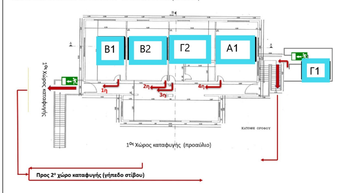
ΣΧΕΔΙΟ ΕΚΚΕΝΩΣΗΣ ΚΤΗΡΙΟΥ ΓΕΛ ΛΕΡΟΥ –ΜΠΟΥΛΑΦΕΝΤΕΙΟ (ΟΡΟΦΟΣ)
