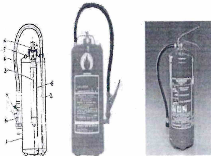
Πυροσβεστήρας ξηράς σκόνης συνεχούς πίεσης
