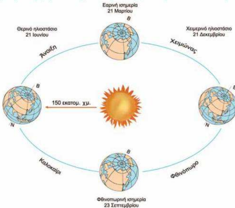
Εικόνα 5.1: Οι κινήσεις της Γης
