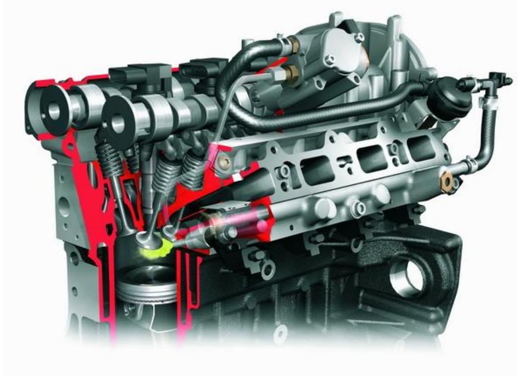
4χρονος βενζινοκινητήρας τη στιγμή της έκχυσης βενζίνης
