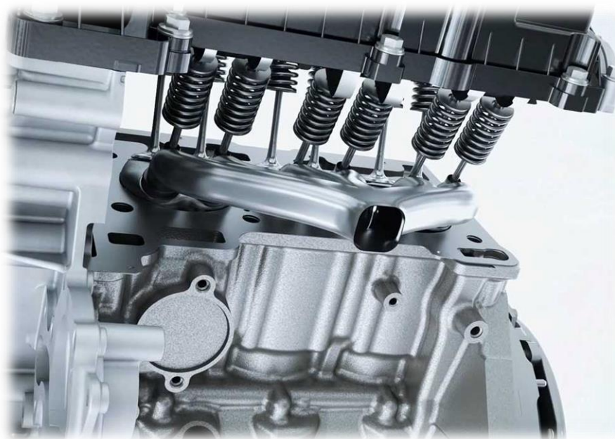
4χρονος βενζινοκινητήρας Ford Ecoboost
