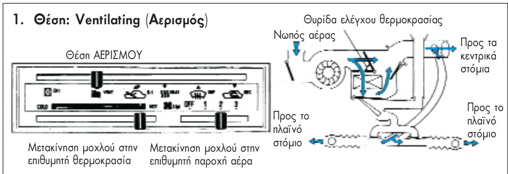
Σχ.8.9 Ροή αέρα κατά τον αερισμό (ρομπινέτο καλοριφέρ κλειστό).
