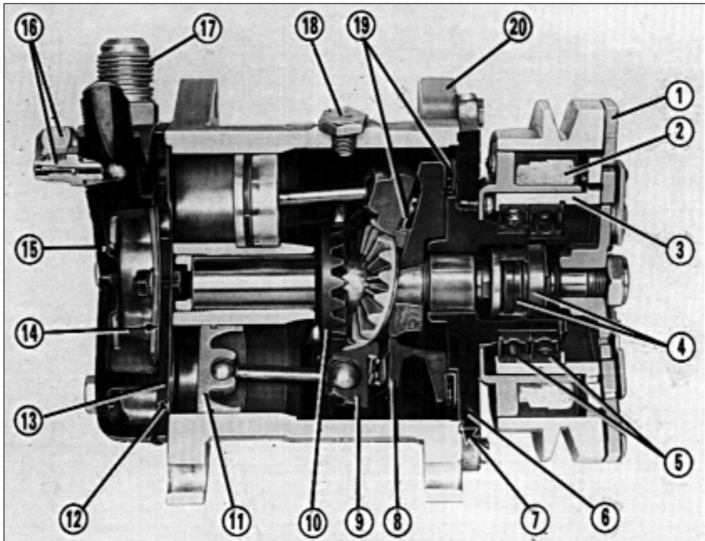
Σχ.8.19 Διαμήκης τομή περιστροφικού συμπιεστή
