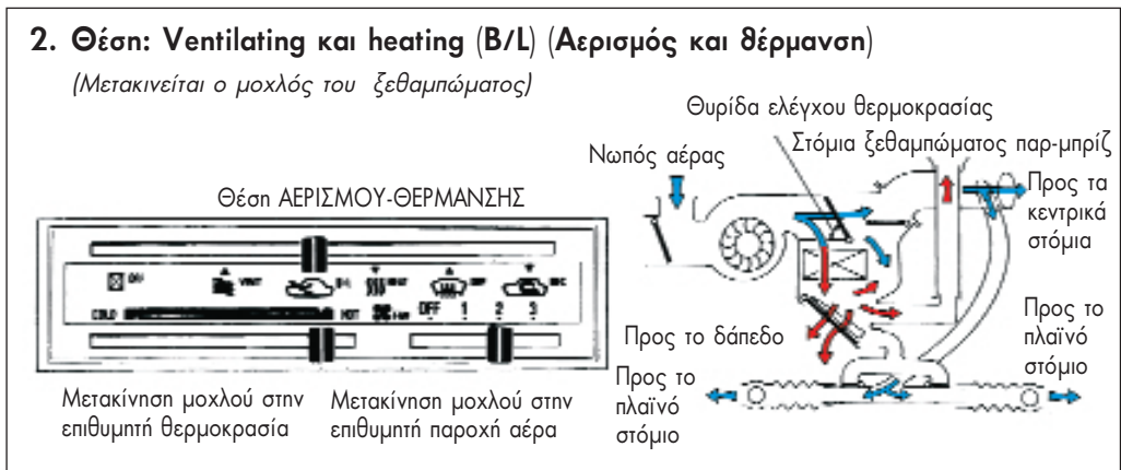
Σχ.8.10 Ροή αέρα κατά τον αερισμό και θέρμανση
