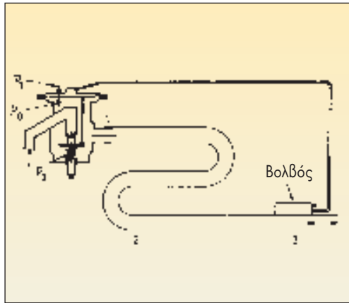
Σχ. 8.25 Σχηματική διάταξη αρχής λειτουργίας θερμοστατικής βαλβίδας: Ρο πίεση ατμοποίησης, Ρ1 πίεση βολβού (αισθητηρίου), Ρ3 πίεση ελατηρίου.
