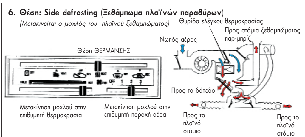
Σχ.8.14 Ροή αέρα κατά το ξεθάμπωμα του παρ-μπριζ και των πλαινών παραθύρων οδηγού και συνοδηγού (με επιλογή παράλληλης θέρμανσης του αέρα).
