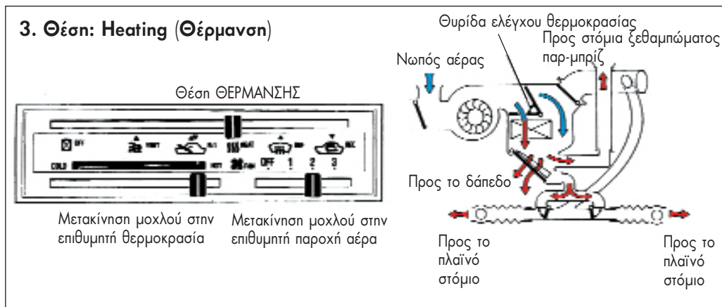
Σχ.8.11 Ροή αέρα κατά τη θέρμανση
