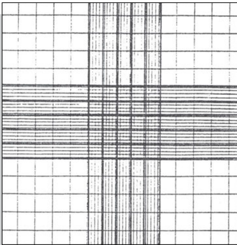
Σχήμα 15.2 Περιοχές της πλάκας Neubauer, όπως φαίνονται από το μικροσκόπιο
