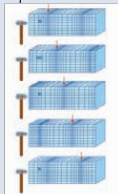
Κύματα P
