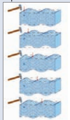
Κύματα S
