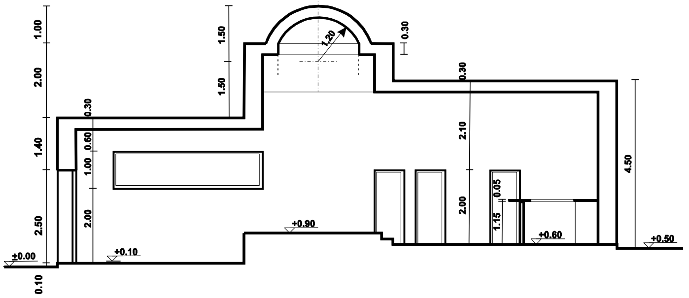
ΤΟΜΗ A-A
