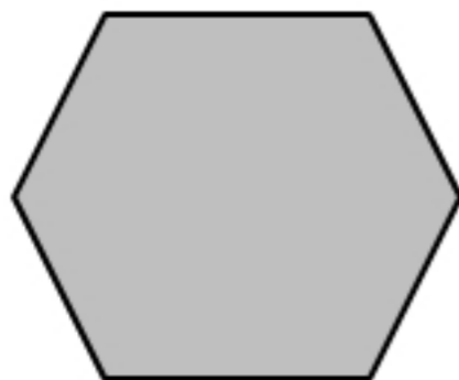
εξάγωνο
