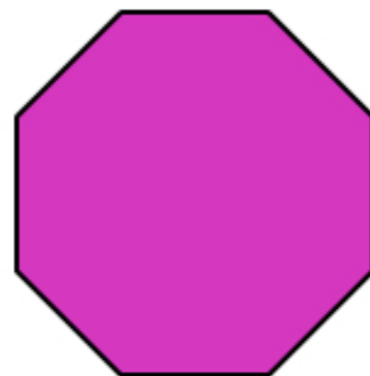
οκτάγωνο
