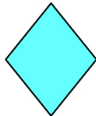
ρόμβος
