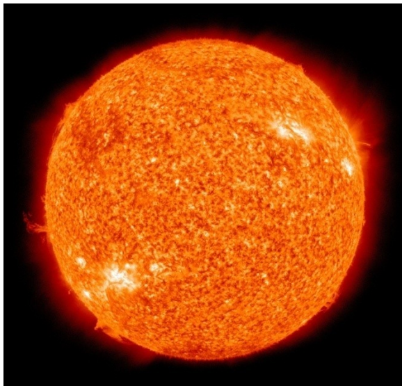
Ήλιος: ένας τεράστιος καυτός αστέρας
