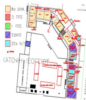
Κάτοψη Ισογείου
