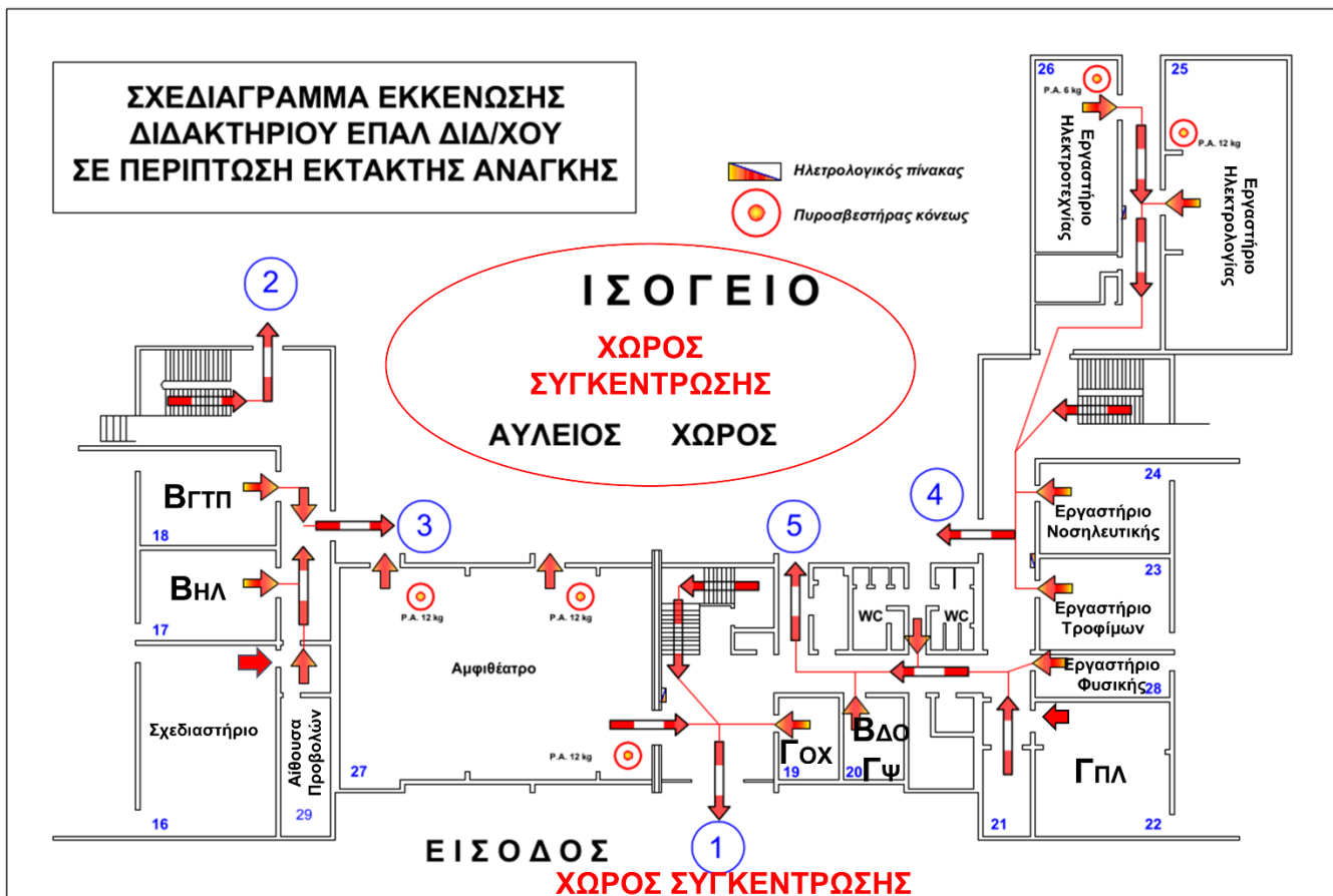
(β) Σχεδιάγραμμα (α) Όροφος (β) Ισόγειο
