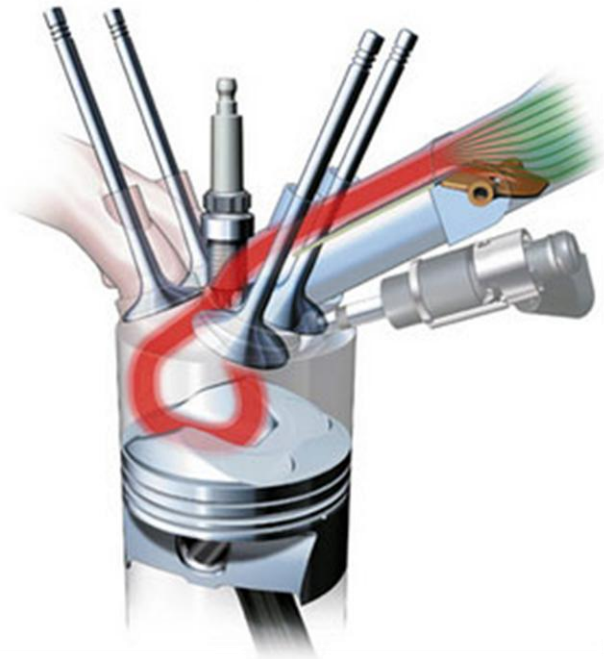
Schichtladebetrieb Stratified-charge operation
